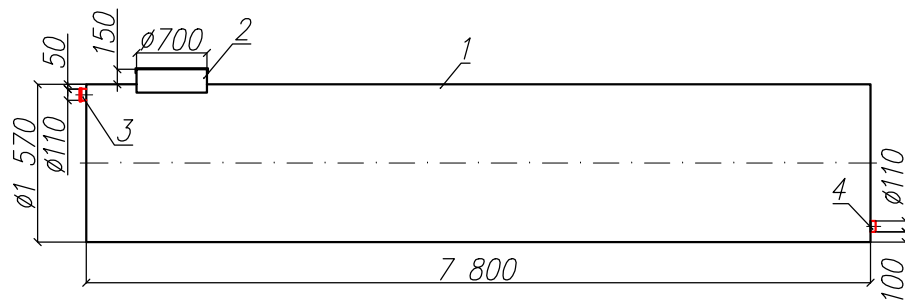
Разрез 1-1
