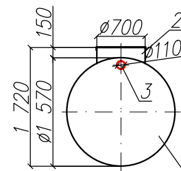
Вид спереди
